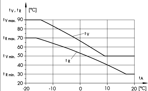
Rys. 5 · Pogodowa regulacja temperatury zasilania z płynnym ograniczeniem temperatury wody powrotnej
