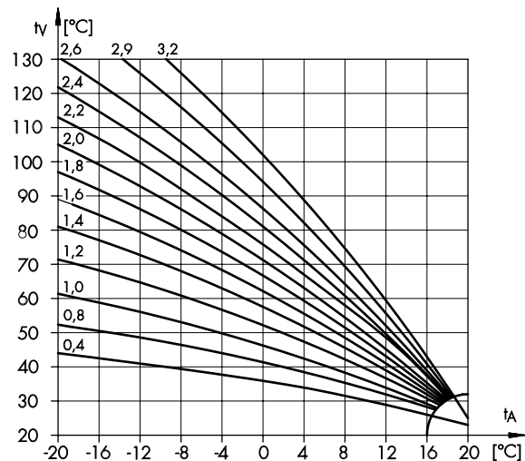
Rys. 4 · Krzywe grzania
