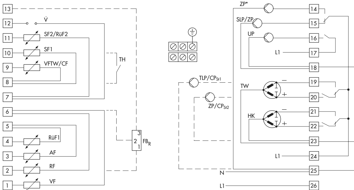
Rys. 9 · Przyporządkowanie zacisków
