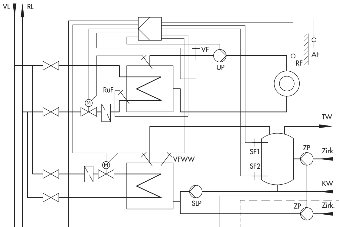
Rys. 8 · Schemat instalacji 5.0
