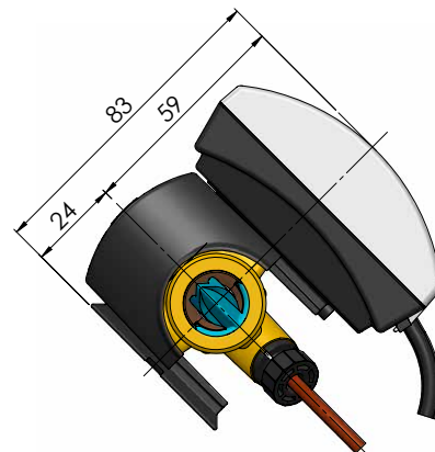
MULTICAL® 302 z przelicznikiem montowanym na przetworniku przepływu
