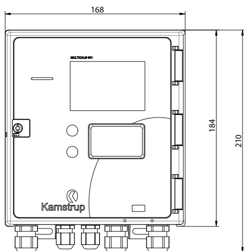
Wymiary zewnętrzne MULTICAL® 801
