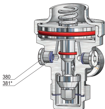
Manometerbohrung G 1/4
