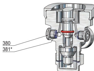
Manometerbohrung G 1/4
