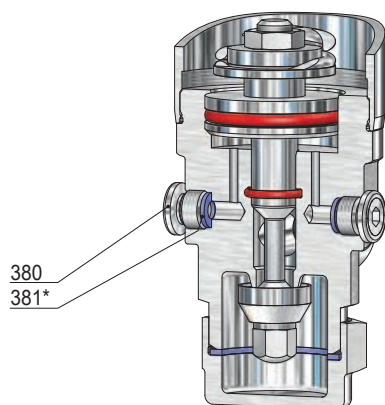
Manometerbohrung G 1/4
