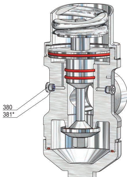
Manometerbohrung G 1/4
